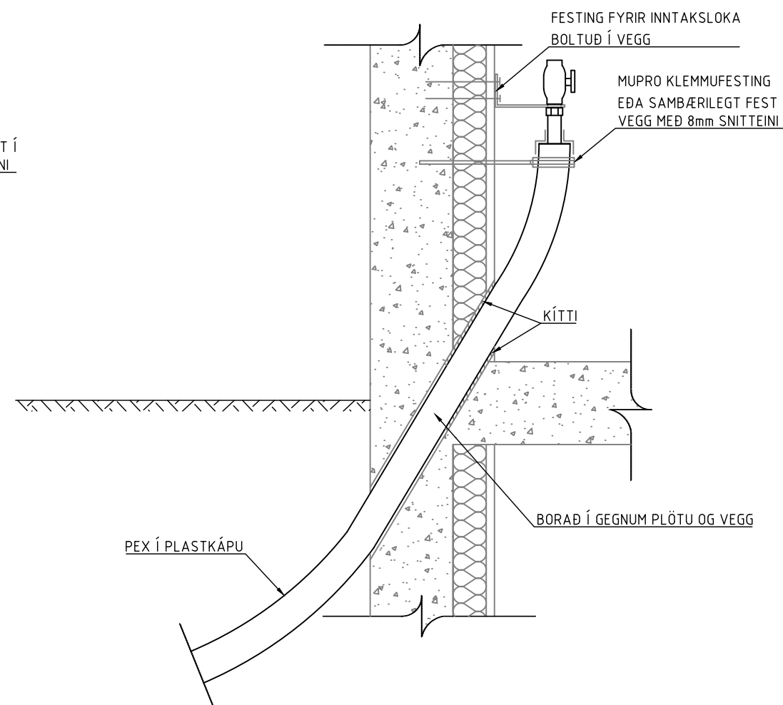
NR.6 – BORADÐ GEGNUM PLÖTU OG VEGG
