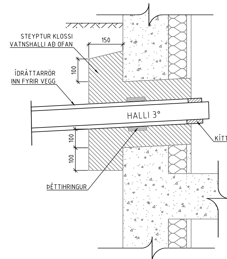
NR.3 - BROTIÐ OG MEÐ KLOSSA
