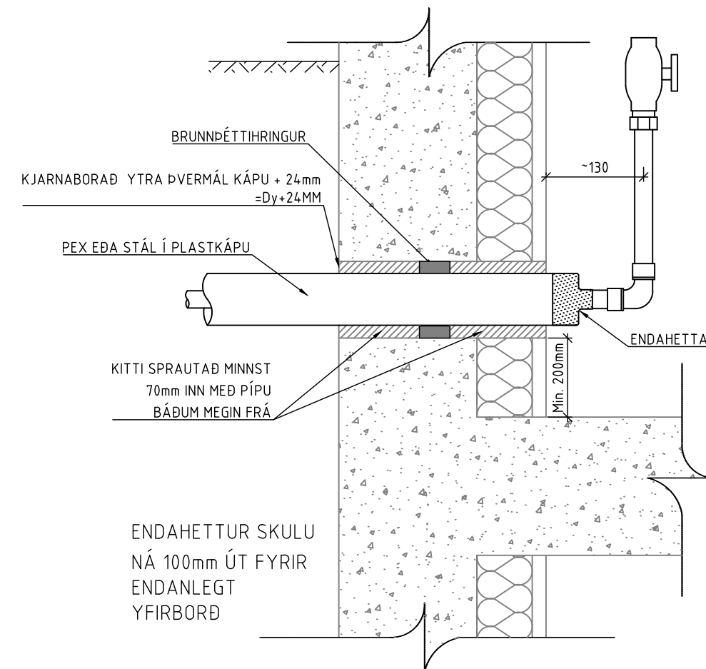
NR.2 – INN ÚR VEGG (KJARNABORÐ 90°)
