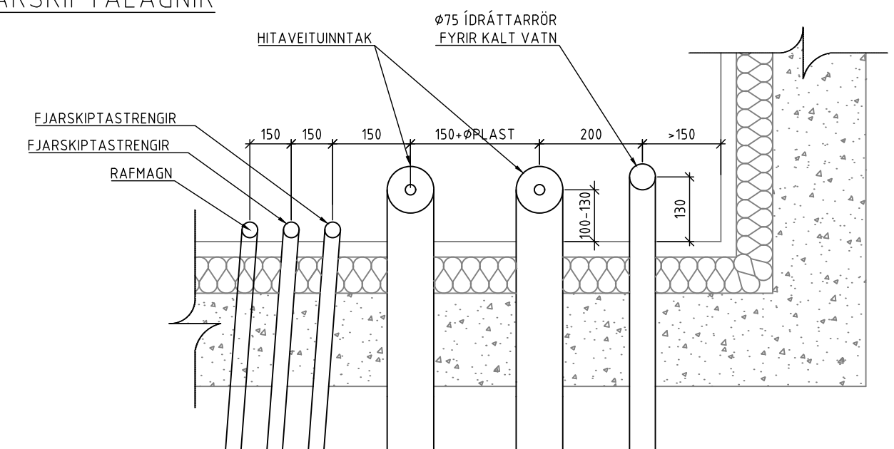
NR.7 - GRUNNMYND: INNTÖK HS VEITUR OG FJARSKIPTALAGNIR
