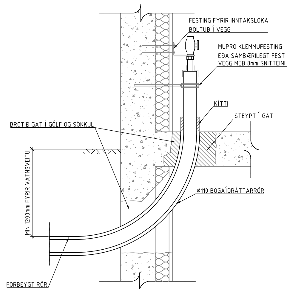
NR.5 – UPP ÚR GÓLFI (ÍDRÁTTARRÖR)
