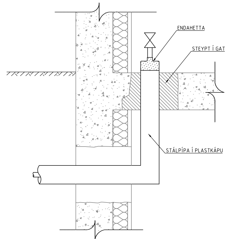
NR.5 – UPP ÚR GÓLFI (ÍDRÁTTARRÖR)
